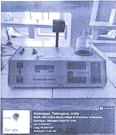
KARLFISCHER TITRIMETER
