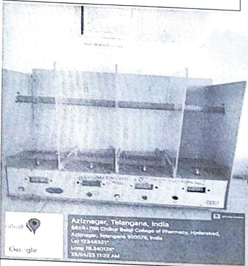
ROTAROD APPARATUS
